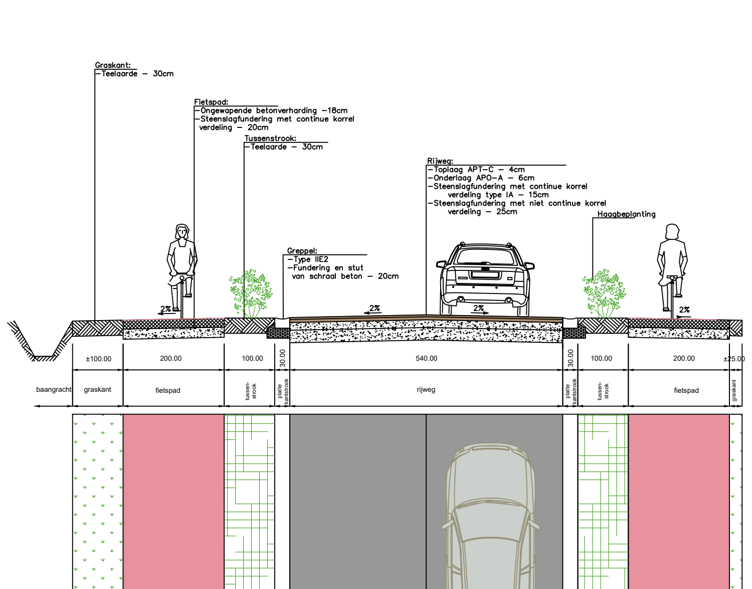
TYPEDWARSPROFIEL 3
