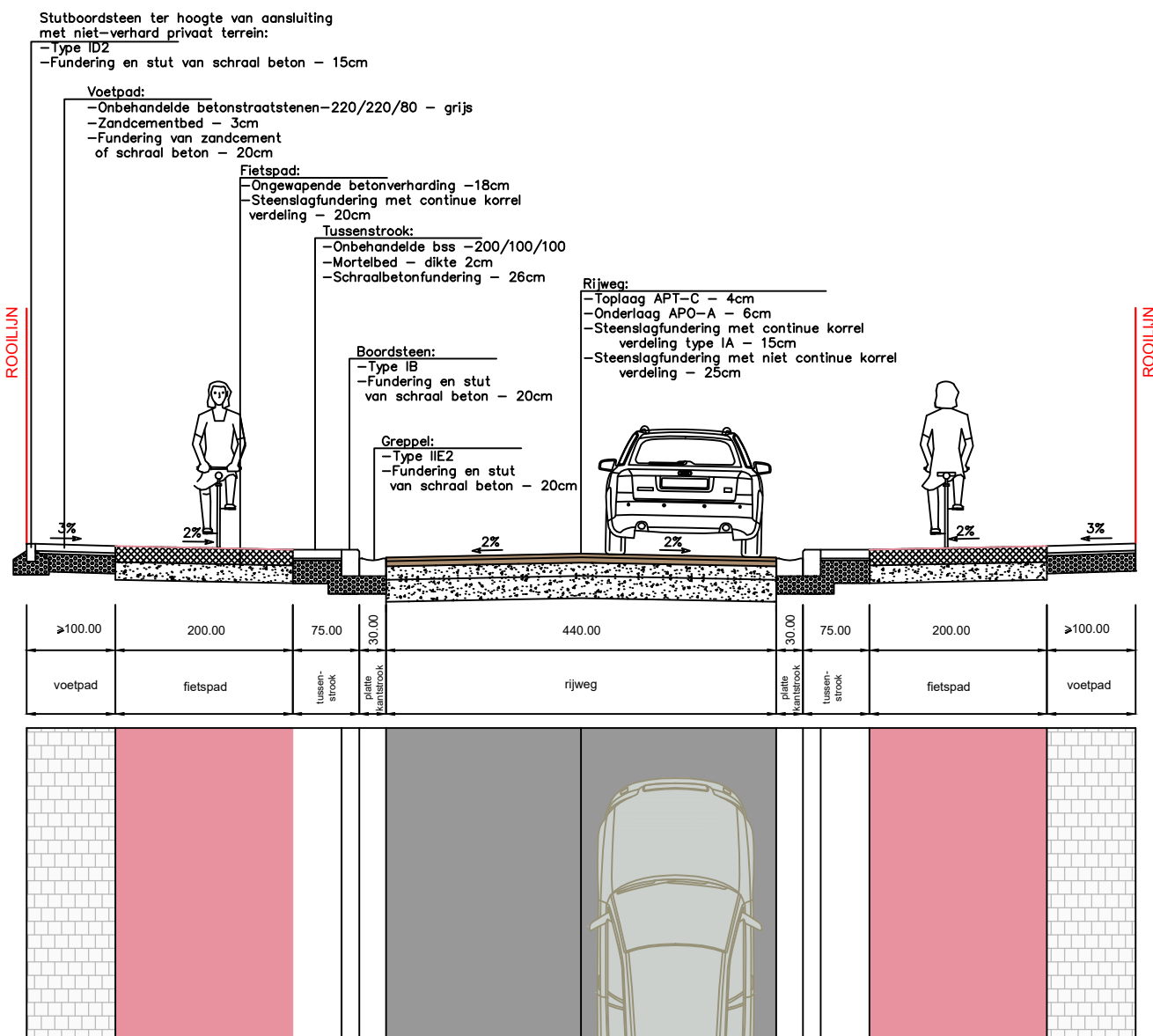
TYPEDWARSPROFIEL 1
