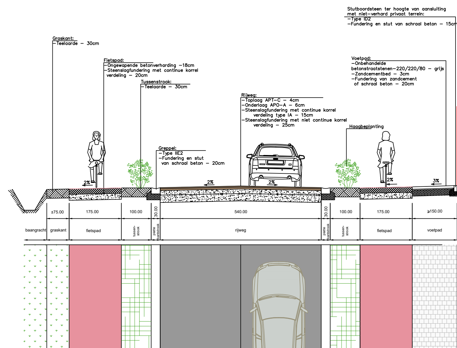
TYPEDWARSPROFIEL 5
