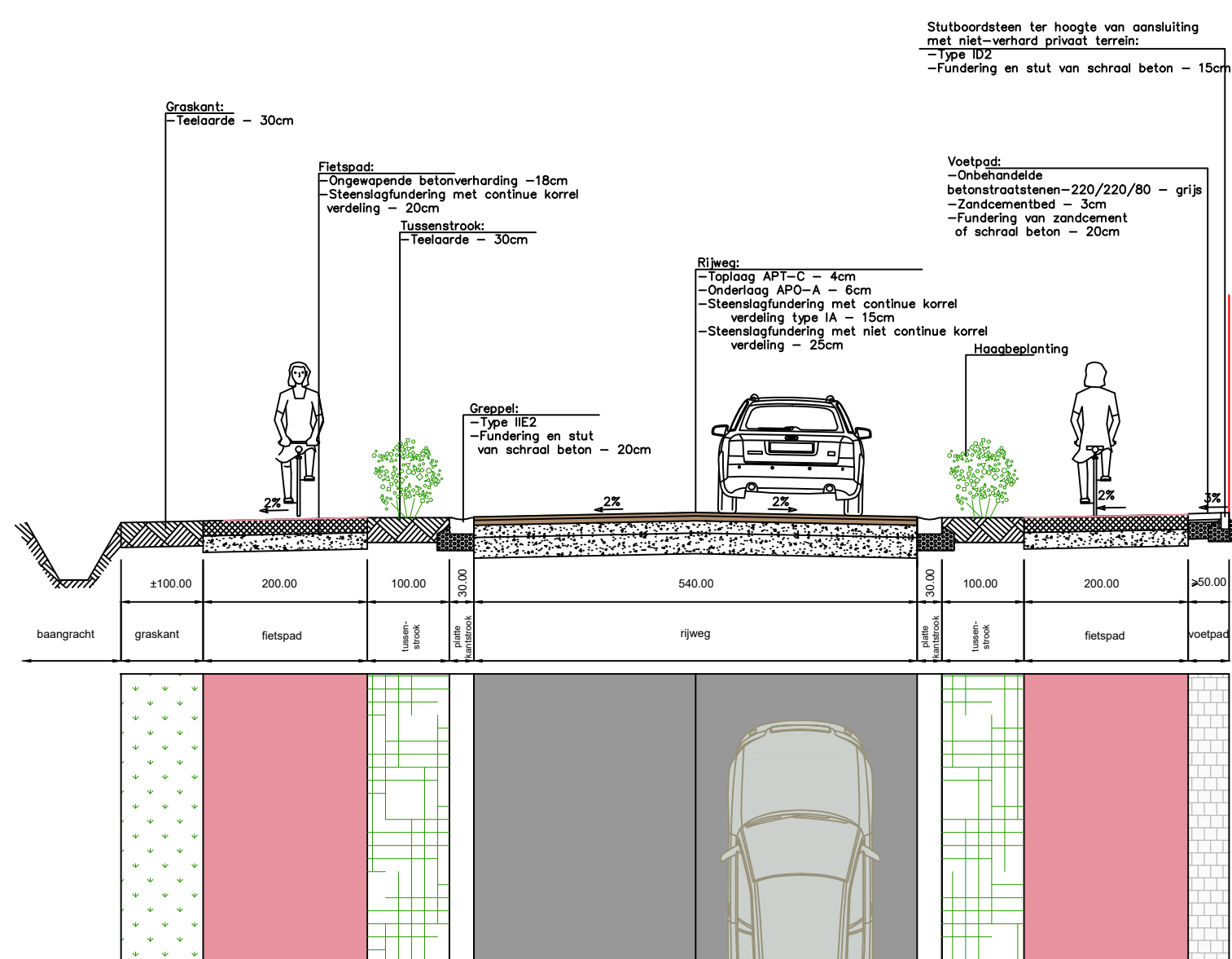
TYPEDWARSPROFIEL 2
