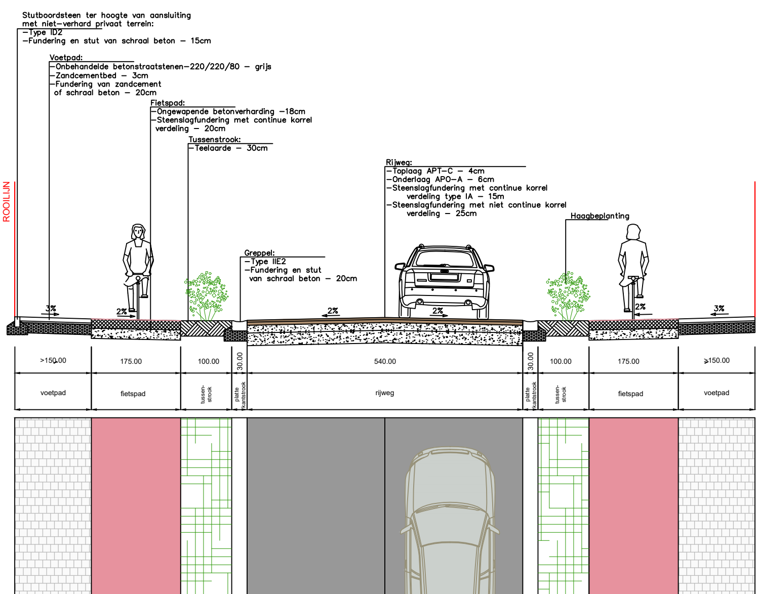
TYPEDWARSPROFIEL 4
